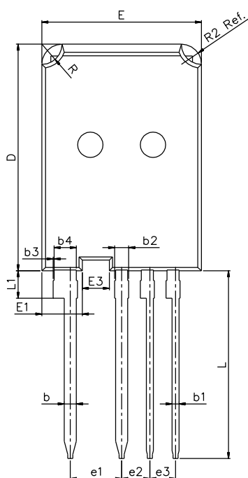
TO-247P-4L
