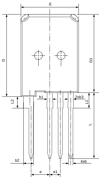
TO-247P-4L
