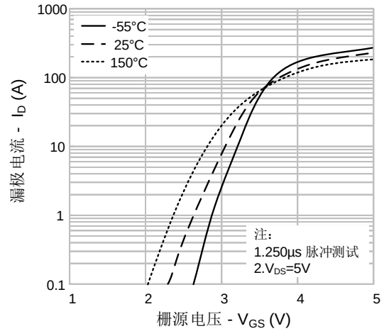
图 2. 传输特性
